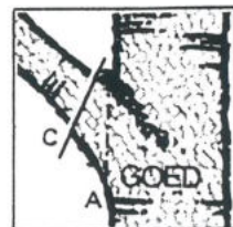
Zaagsnede begint aan de takzijde van takschorsrichel hoek A-B is gelijk aan hoek A-C. Stippellijn is denkbeeldige lijn langs de stam.
