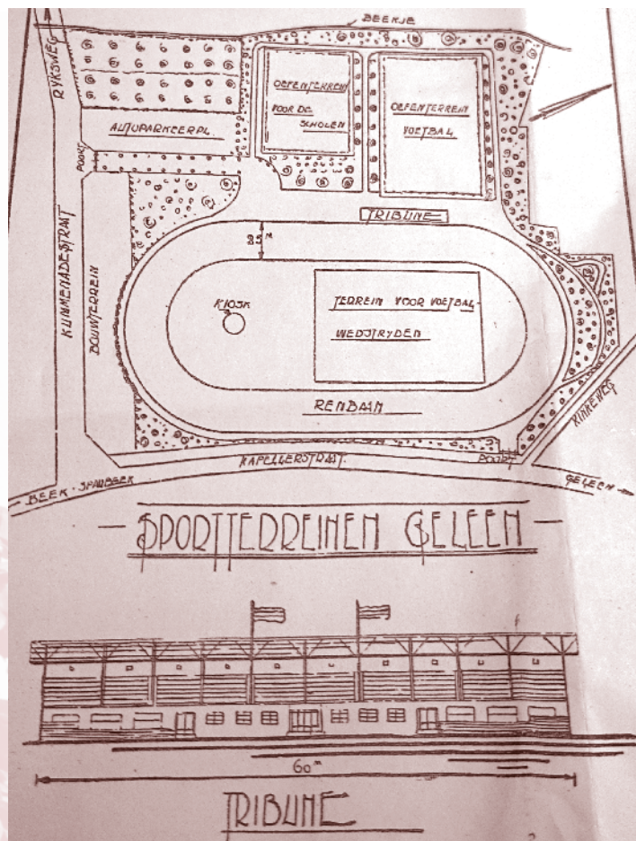
Ontwerptekening van het Sportpark in Geleen (Bron: Archief De Domijnen)
